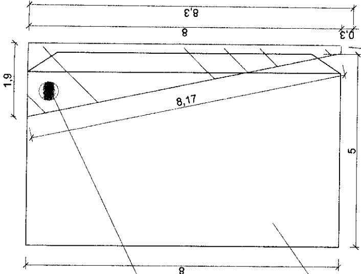
Tampa frontal em acrílico transparente 2 mm (Para proteção do acionador manual)
